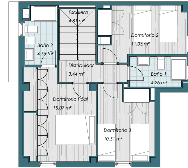
PLANTA PRIMERA
